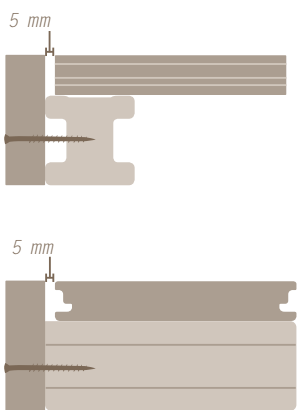
Abschlussleiste mit MYDECK Dielen [Abb. 16]
