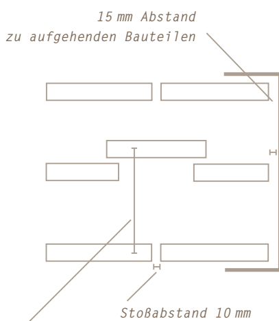
UNTERKONSTRUKTION [40 cm Mittenabstand] Für ein einheitliches Schraubenbild bei sichtbarer Verschraubung Unterkonstruktion nicht versetzt.
