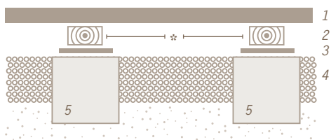
Verlegung auf verdichtetem Schotter [Abb. 3]
